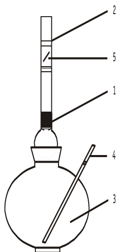
Bild 1 Gasoszillator
