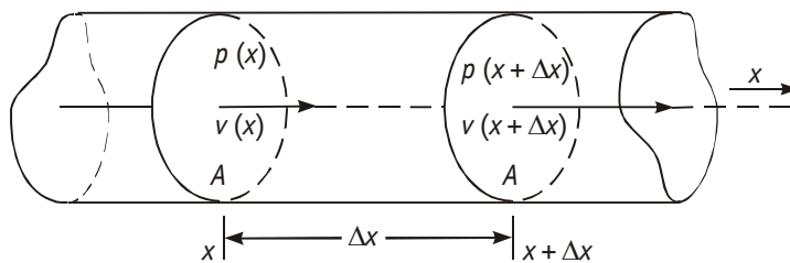
Bild 1 Zur Herleitung der Wellengleichung
