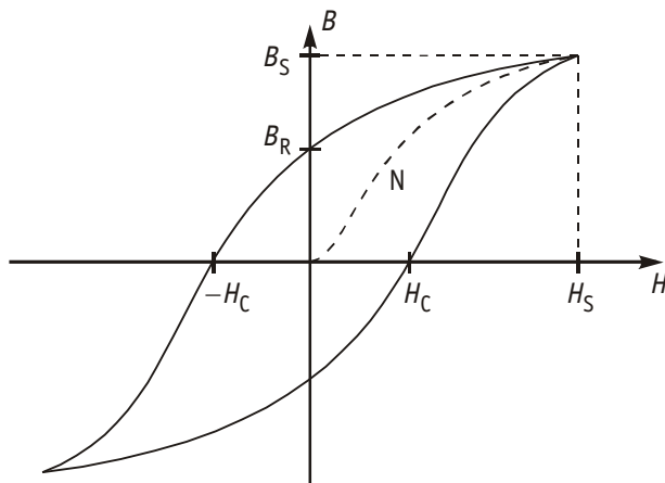
Bild 1 Hystereseschleife
